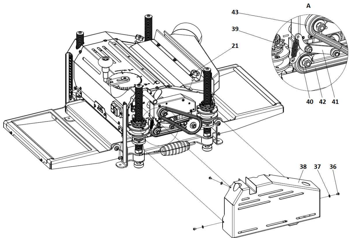
Рисунок 7. Цепная передача
